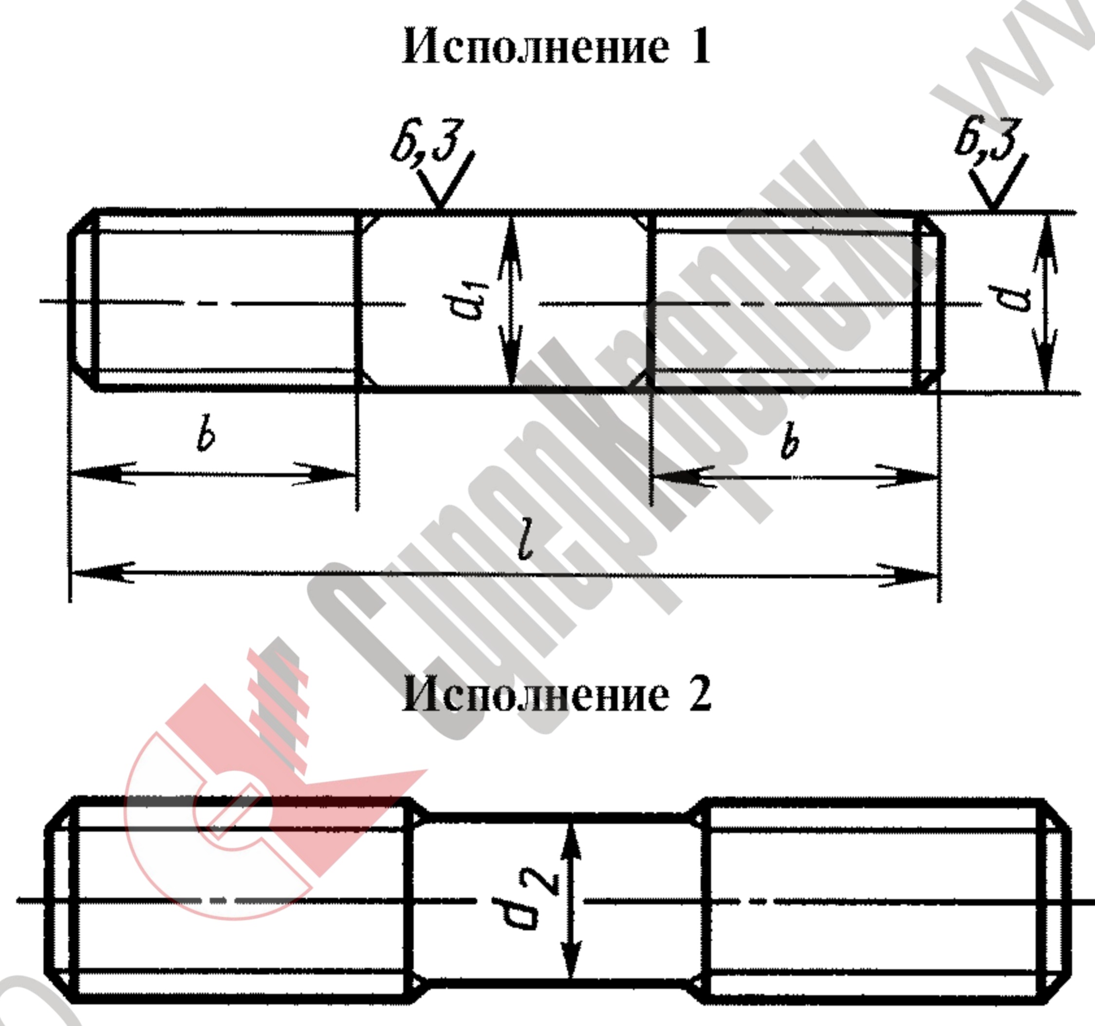
d_2 приблизительно равен среднему диаметру резьбы
