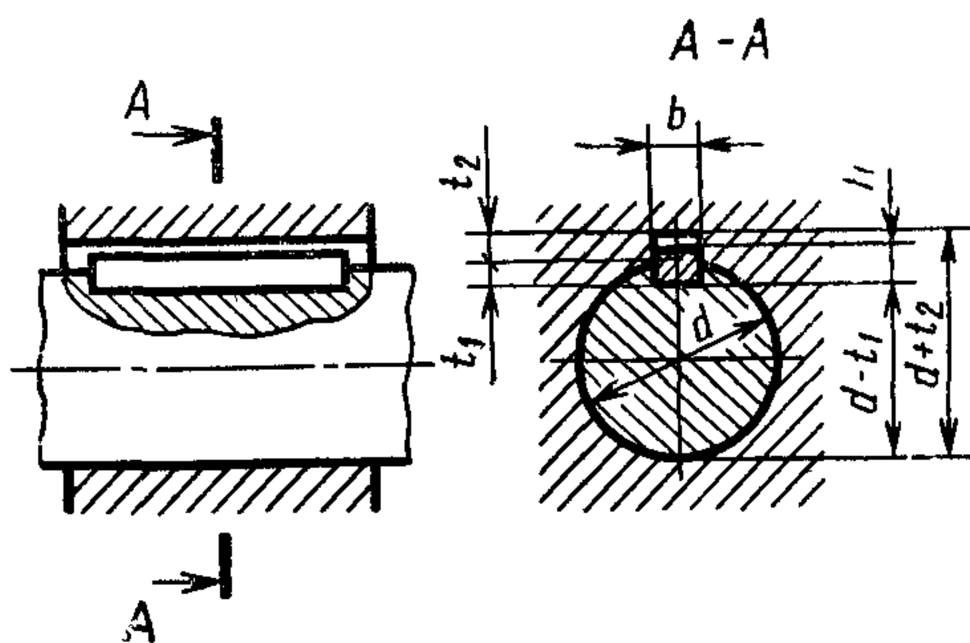
Шпоночные пазы вала и втулки
